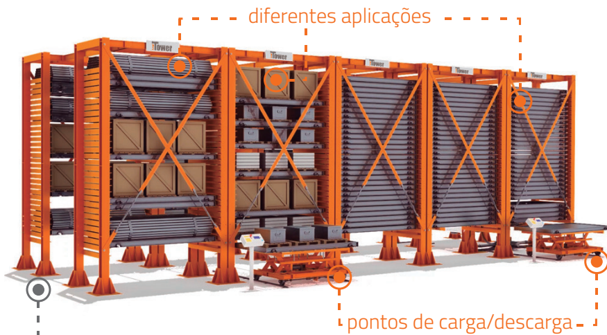
MULTI LOGITOWER ARMAZENAGEM EM COLUNAS MÚLTIPLAS
